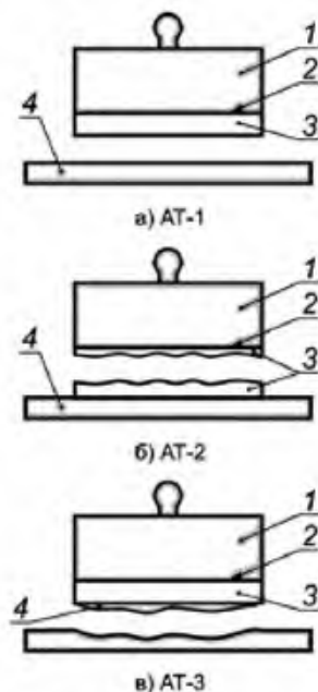
1 — стальная пластина; 2 — эпоксидный клей; 3 — образцы пены; 4 — основание
