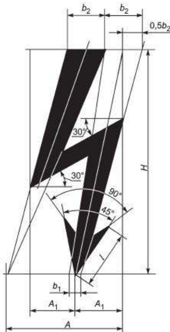
Рисунок Н.1 - Графический символ электрического напряжения
