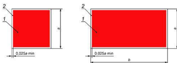
Рисунок 4 - Основа цветографического изображения и соотношение размеров знаков пожарной безопасности
