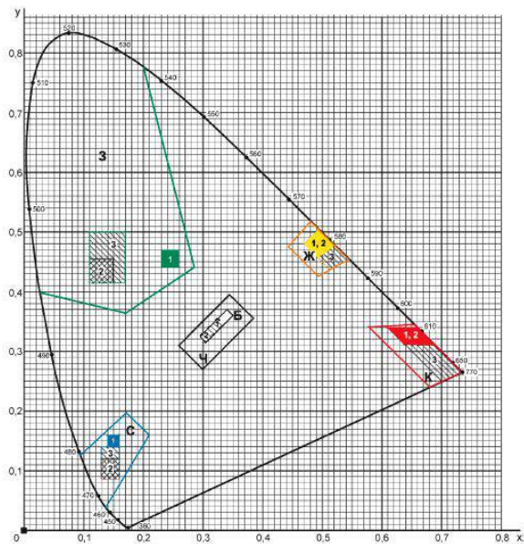
Рисунок А.1 - Допустимые области цветности x, y сигнальных и контрастных цветов на стандартном цветовом графике МКО 1931 г.
