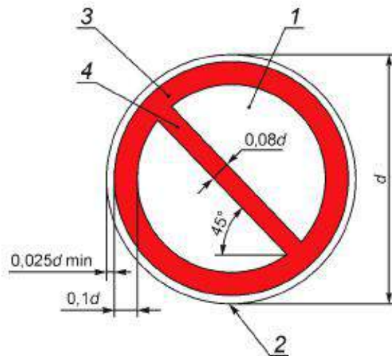
Рисунок 1 - Основа цветографического изображения и соотношение размеров запрещающих знаков безопасности
