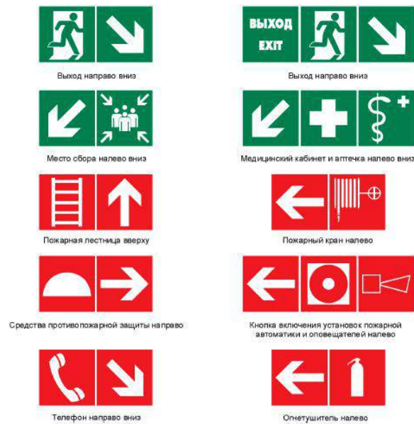
Рисунок 10 - Примеры формирования смысловой комбинации знаков для указания направления движения к эвакуационному выходу, средствам противопожарной защиты, месту сбора и средствам оказания первой медицинской помощи
