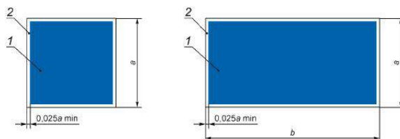
Рисунок 6 - Основа цветографического изображения и соотношение размеров указательных знаков безопасности
