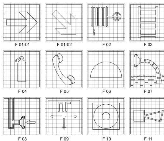
Рисунок П.4 - Знаки пожарной безопасности
