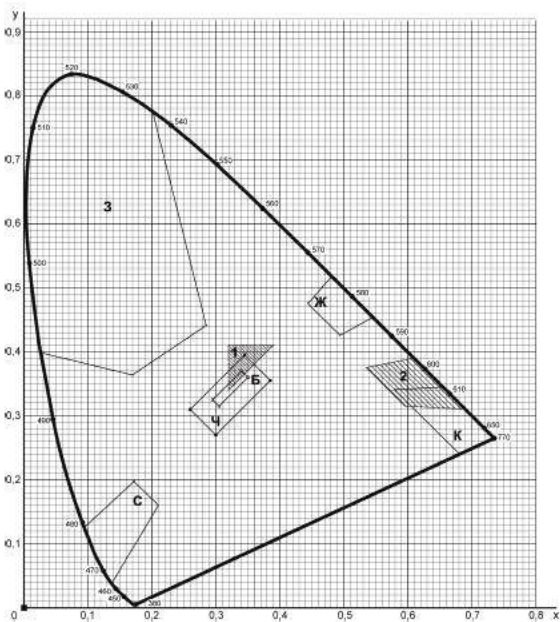
Рисунок Б.1 - Допустимые области цветности сигнальных и контрастных цветов фотолюминесцентных материалов на стандартном цветовом графике x, y МКО 1931 г.
